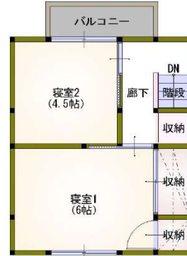
〔2階 平面図〕
