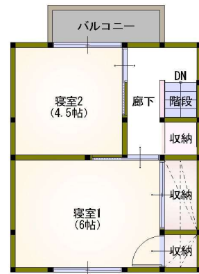
〔2階 平面図〕
