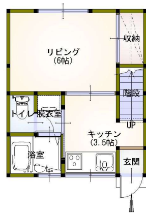
〔1階 平面図〕
